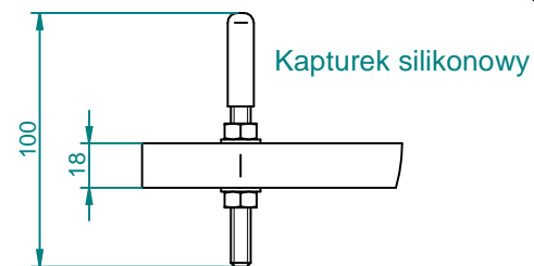
Szczegół A
