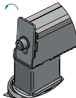
Szczegół A Chowane zabezpieczenie
