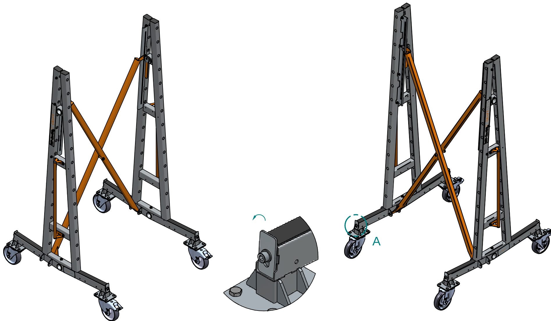
Szczegół A Chowane zabezpieczenie
